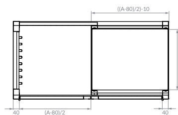
WYMIAR PÓŁKI
