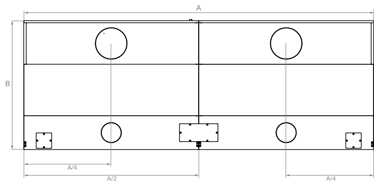
RZUT Z GÓRY
