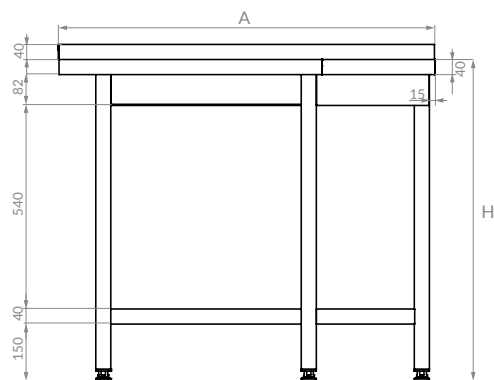
RZUT Z PRZODU
