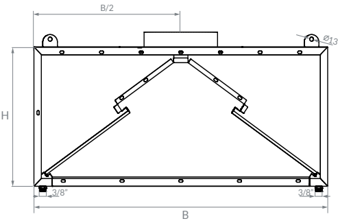
RZUT Z BOKU
