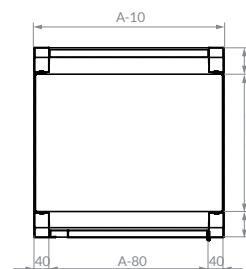
WYMIAR PÓŁKI
