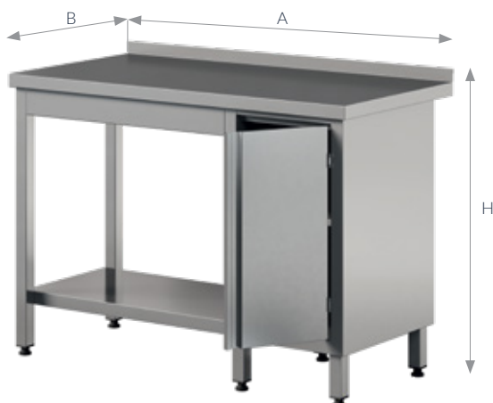
WT-116 PL HD S
