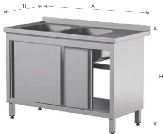
STW-126/2 PL L 2SD
