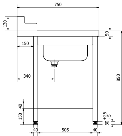
RZUT Z BOKU
