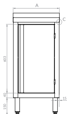
RZUT Z PRZODU
