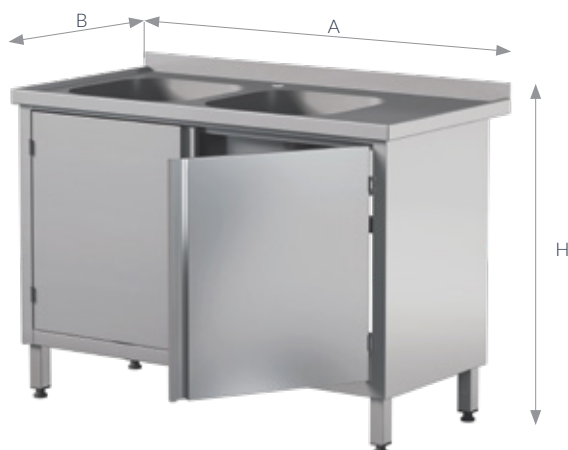
STW-126/2 PL L 2HD C
