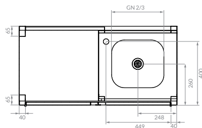
PRZEKRÓJ - WIDOK Z GÓRY
